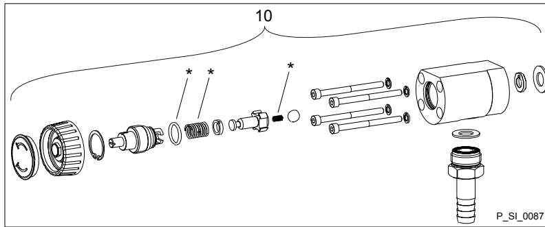
Fig. 34: Sigma/ 2 SSA relief valve-A
